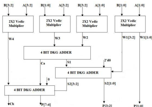
Fig4.10 : 4 Bit Vedic multiplier
