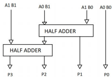
Fig 4.9: 2x2 Vedic multiplier
