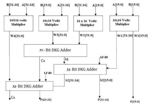
Fig 4.13: 32 Bit Vedic multiplier
