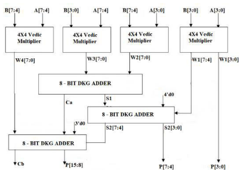
Fig 4.11: 8 Bit Vedic multiplier
