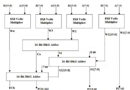
Fig 4.12: 16 Bit Vedic multiplier
