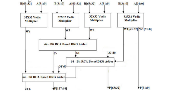
Fig 4.13 64 bit vedic multiplier
